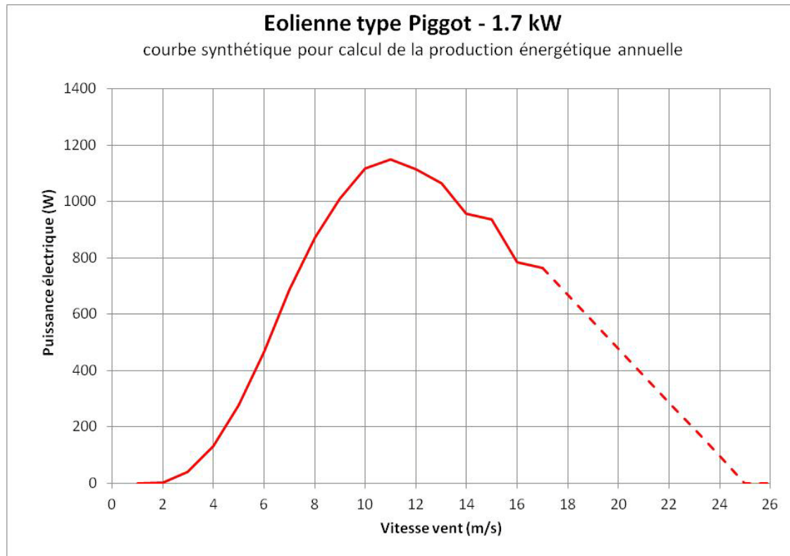
Figure 3-3 Courbe de puissance synthétique pour le calcul de la production énergétique.
