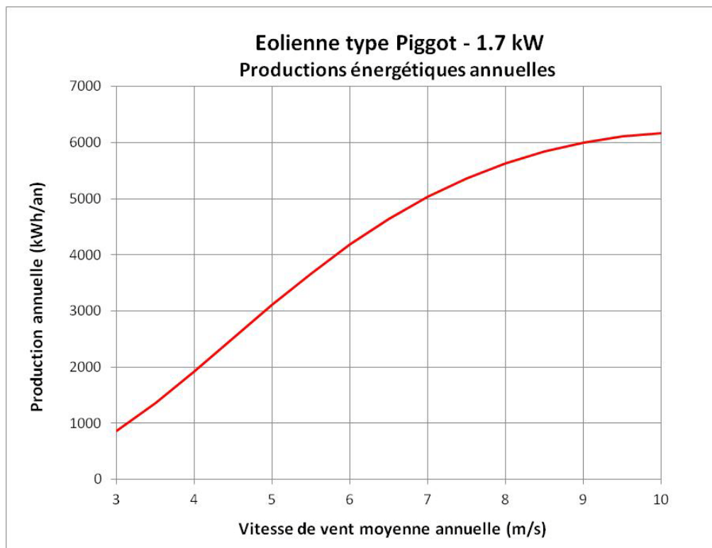
Figure 3-4 Production énergétique annuelle en fonction de la vitesse moyenne annuelle.
