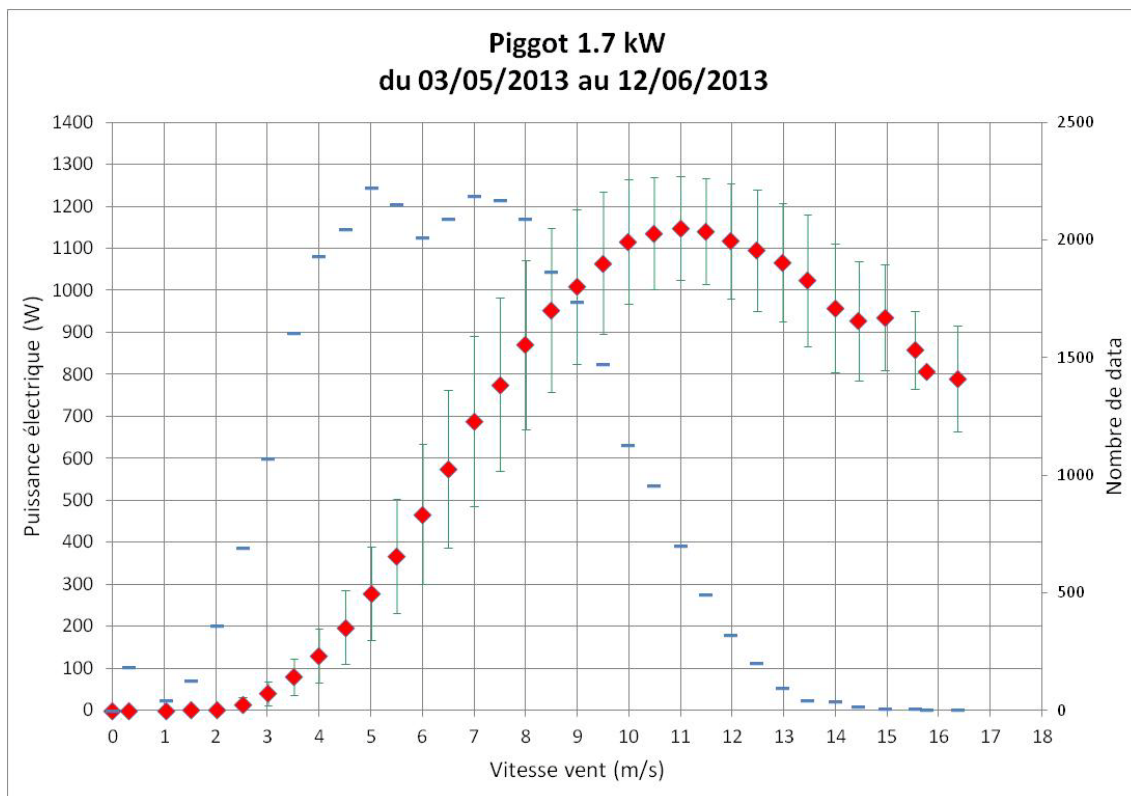
Figure 3-1 Courbe de puissance mesurée sur le site de Malbouissou
