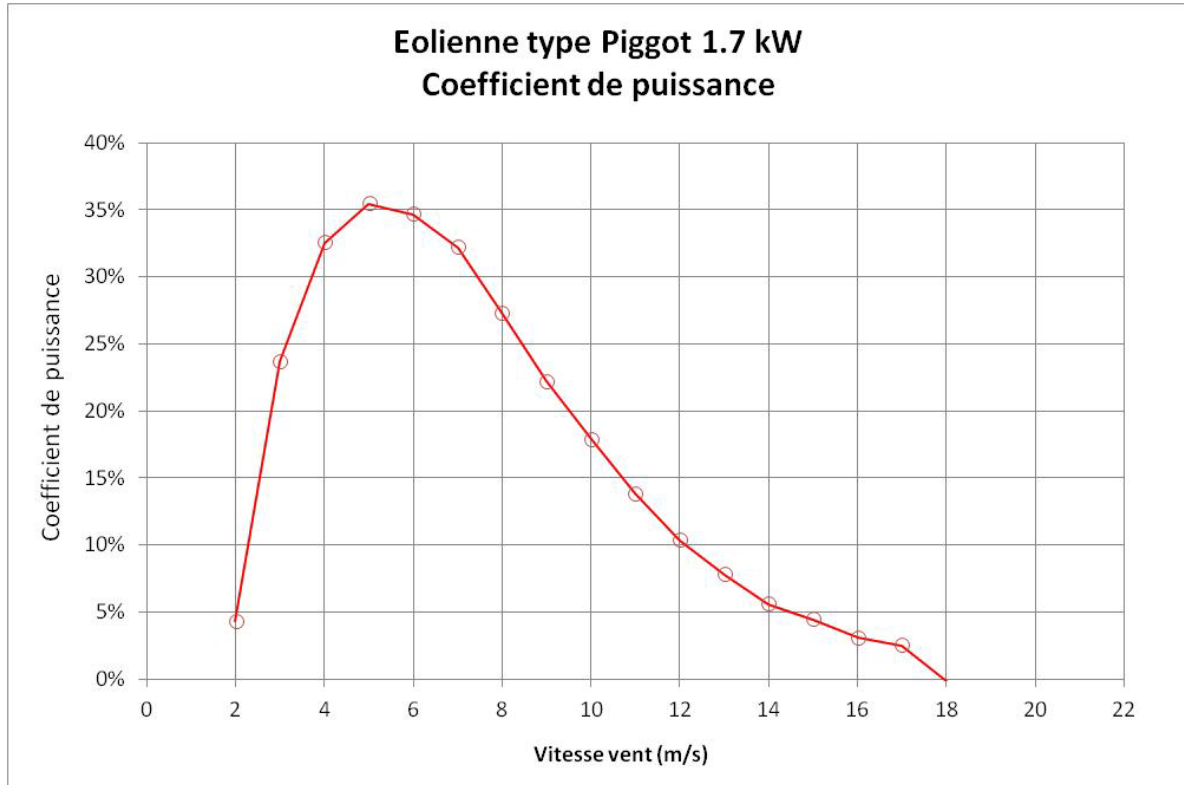
Figure 3-2 Coefficient de puissance
