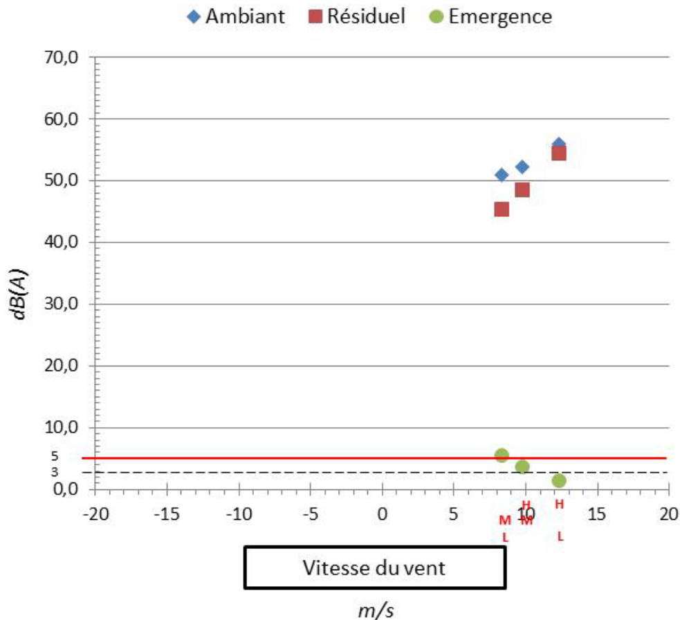
Fiche récapitulative Mât N°1 Bis / Point N°3
